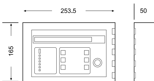
Dimensões dos repetidores ZXr-A e ZXr-P Todas as dimensões em mm.
